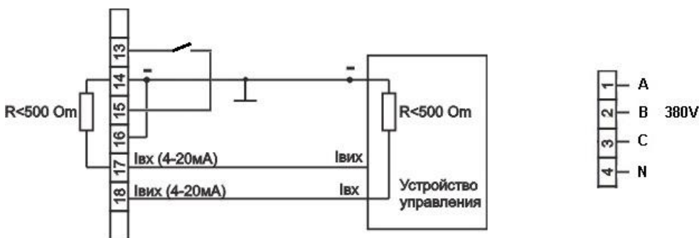
Рис. 2 Схема подключения преобразователя
