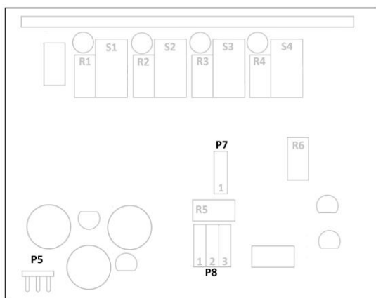
Рис. 1 Расположение регулировочных элементов, плата преобразователя
