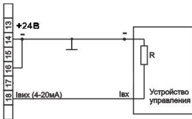
Рис. 2 Схема подключения преобразователя
