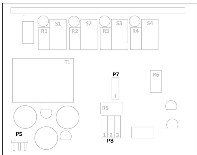
Рис. 1 Расположение регулировочных элементов, плата преобразователя
